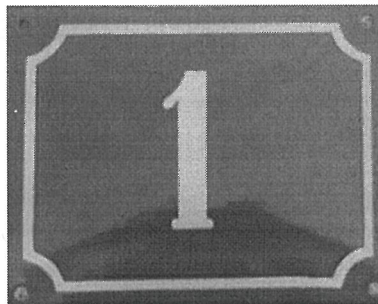
Tabulka orientačního čísla rozměry: 200 X 160 mm velikost arabské číslice: 80 mm
