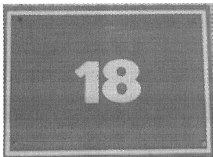
Tabulka evidenčního čísla rozměry: 200 X 150 mm velikost arabské číslice: 40 mm
