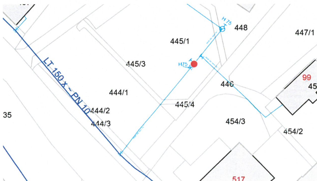
Obrázek 4: Umístění požárního hydrantu na č. parc. 445/1
