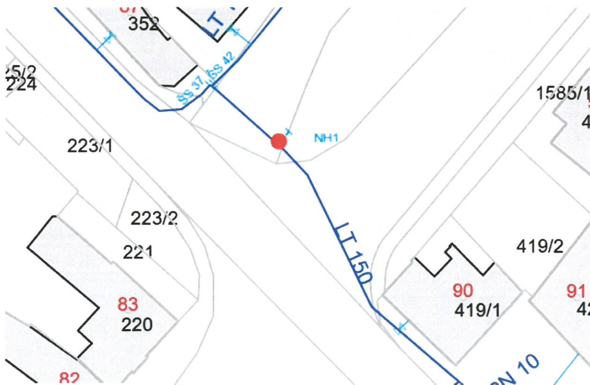
Obrázek 2: Situace umístění požárního hydrantu u č. p. 87 parcelní číslo 417.
