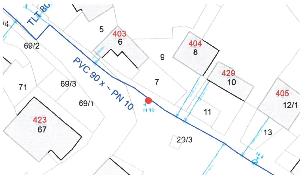
Obrázek 8: Situace umístění nadzemního hydrantu na PVC 90
